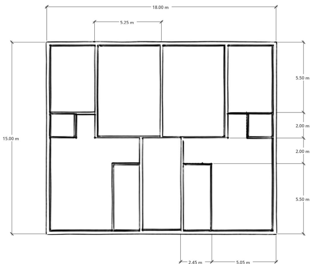
Figur 3. Planvy av en exempelbyggnad
